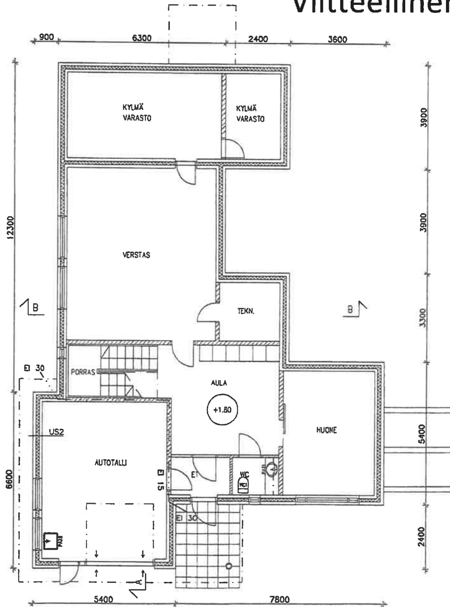
POHJAPIIRROS, KELLARI 1:100
