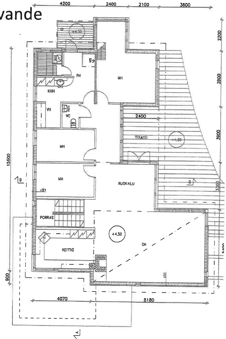
POHJAPIIRROS 1:100
